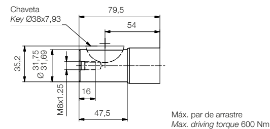
Eje forma H / Shaft form H
