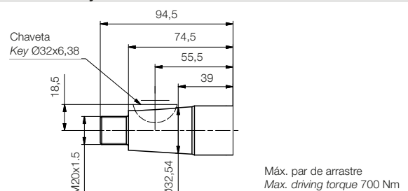
Eje forma J / Shaft form J
