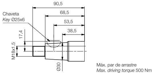
Eje forma A / Shaft form A
