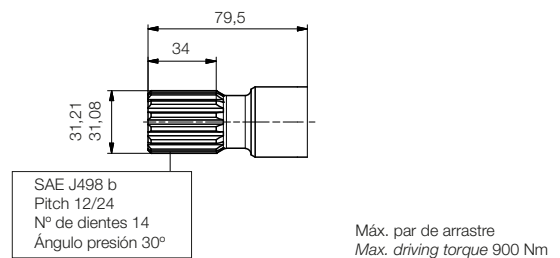
Eje forma J / Shaft form J
