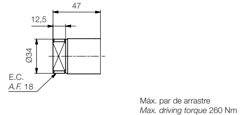
Eje forma B / Shaft form B
